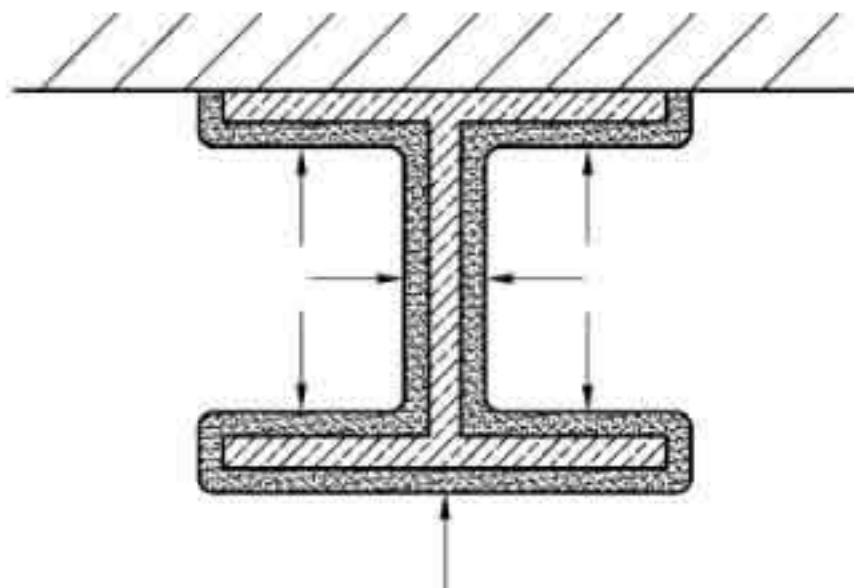
图 1 试件截面上涂层厚度测量点位置
